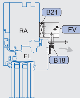
Darstellung am Holz-Fenster
