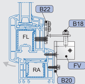
Darstellung am Kunststoff-Fenster
