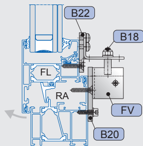
Darstellung am Alu-Fenster
