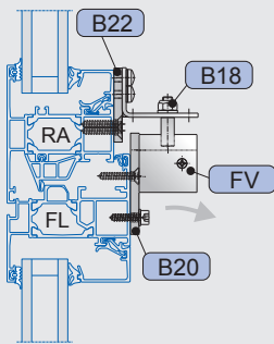
Darstellung am Alu-Fenster
