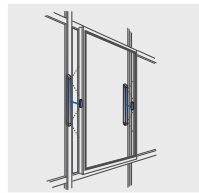
Parallelausstellfenster (PAF)
