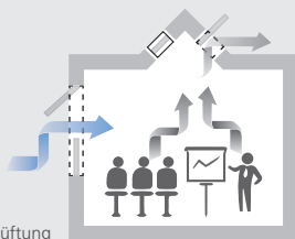
Auftriebslüftung
