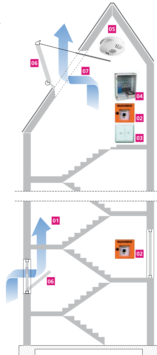
Abb. rechts: Komponenten einer RWA-Anlage
