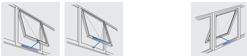
Поворотная створка
