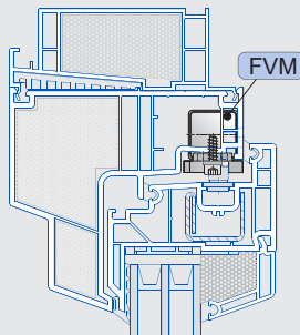
塑料窗
