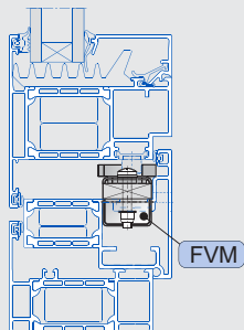
1 隐藏式安装, 外开窗
