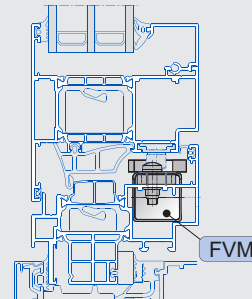
3 隐藏式安装, 外开窗
